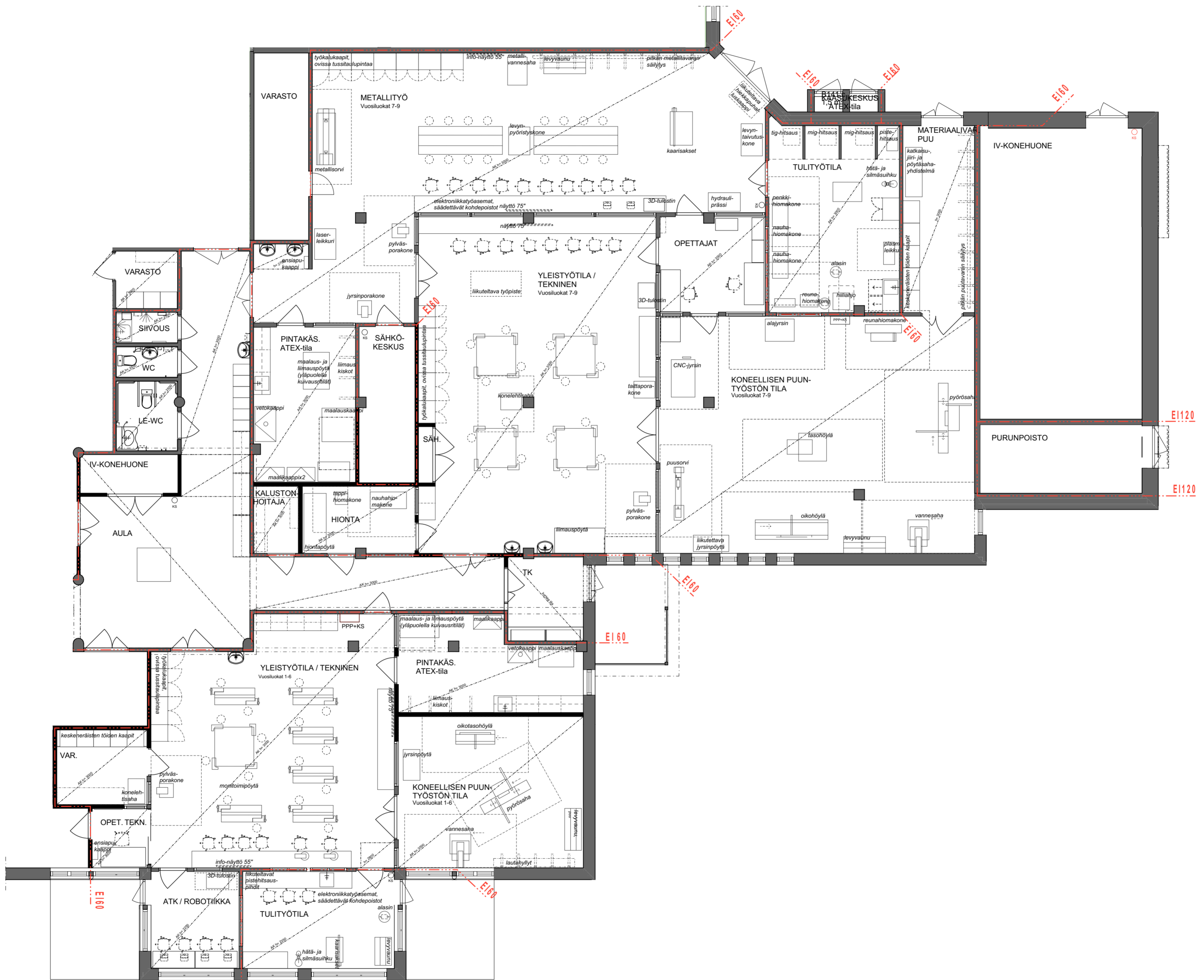
TEKNISEN TYÖN TYÖTAPOJEN TILAT 1:100 (630x594) KOUKKALAN YHTENAIKOULU ARKKITEHTISUUNNITTELU: LINJA ARKKITEHDIT OY / WSP FINLAND OY KUVANKÄSITTELY: OPETUSHALLITUS 2023
